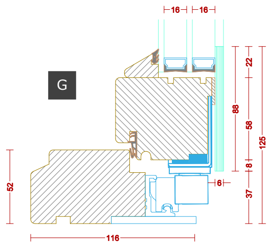
Senkrechter Schnitt
