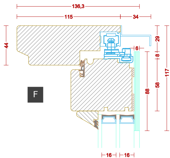
Senkrechter Schnitt
